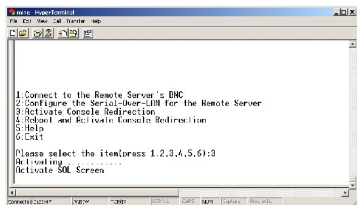
図 3-20. コンソールリダイレクトの例
